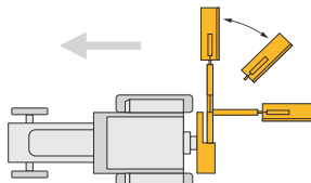
Rotación Hidráulica con dispositivo de seguridad.
